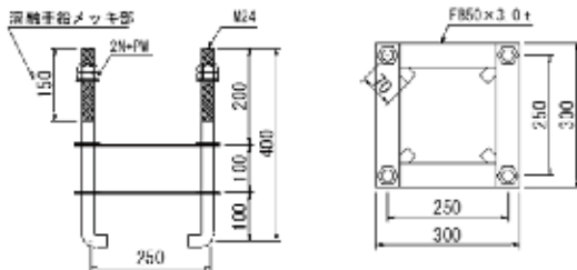
アンカーボルト (例)
