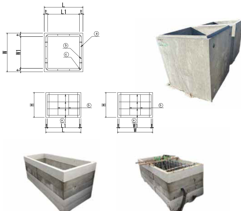
従来の基礎と基礎型枠の工期比較
