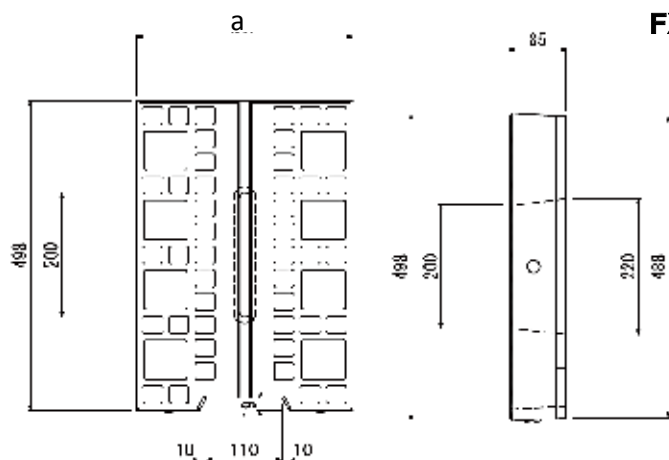
FX側溝 + FX側溝スリット蓋
