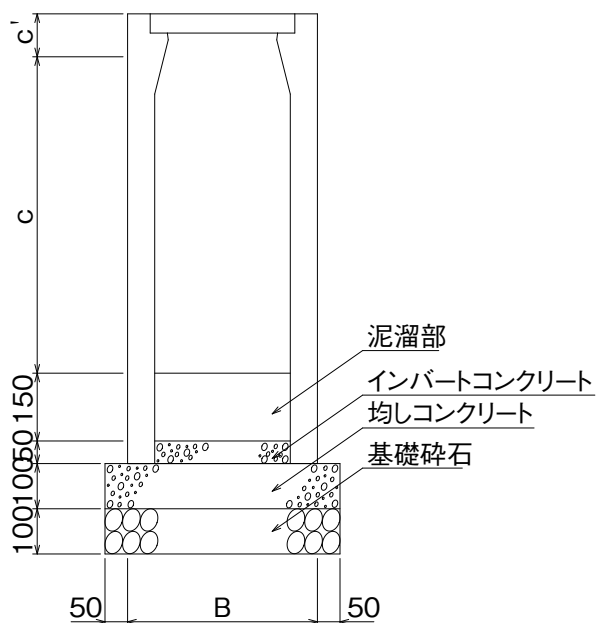
標準断面図
