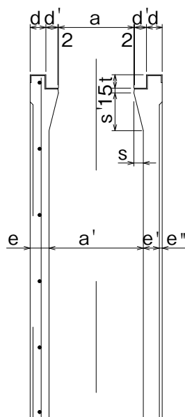
A-A'断面
