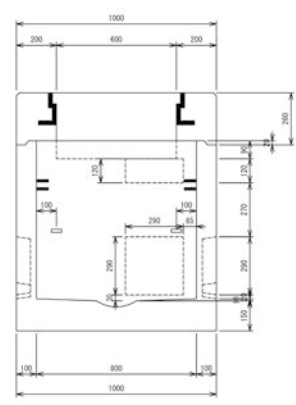
A-A断面図
