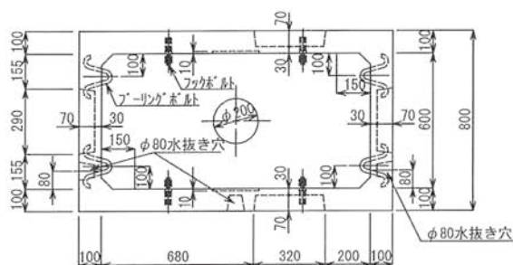
〈CD型〉 重量：1220kg
