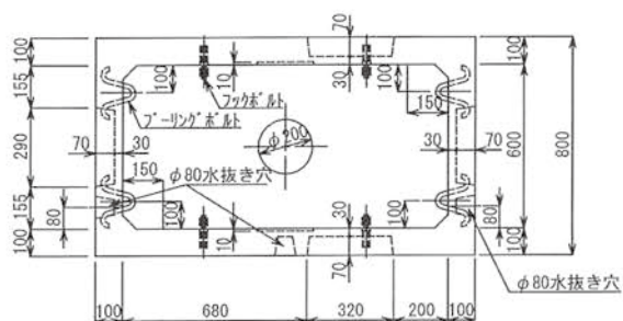
〈CD型〉 重量：1220kg
