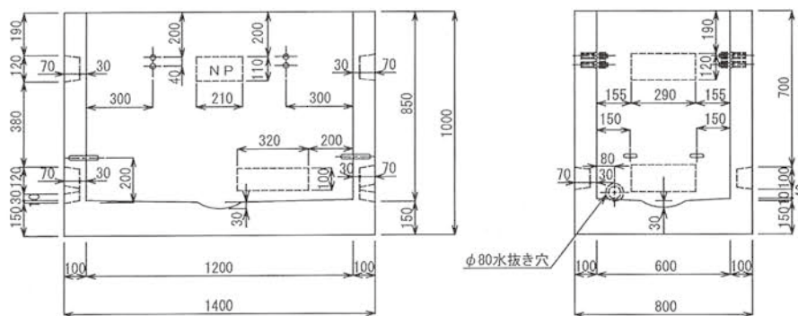
〈CD型〉 重量：1220kg
