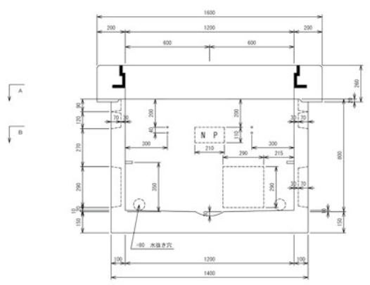
B-B断面図
