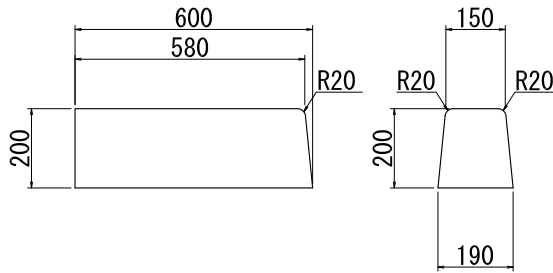
コンビニブロックA 端部
