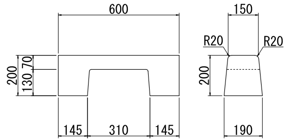
コンビニブロックA 水抜き
