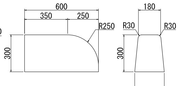
コンビニブロックC 端部
