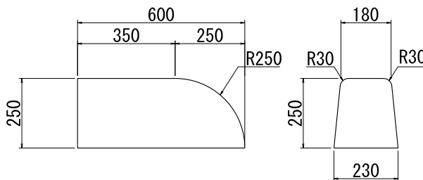
コンビニブロックB 端部
