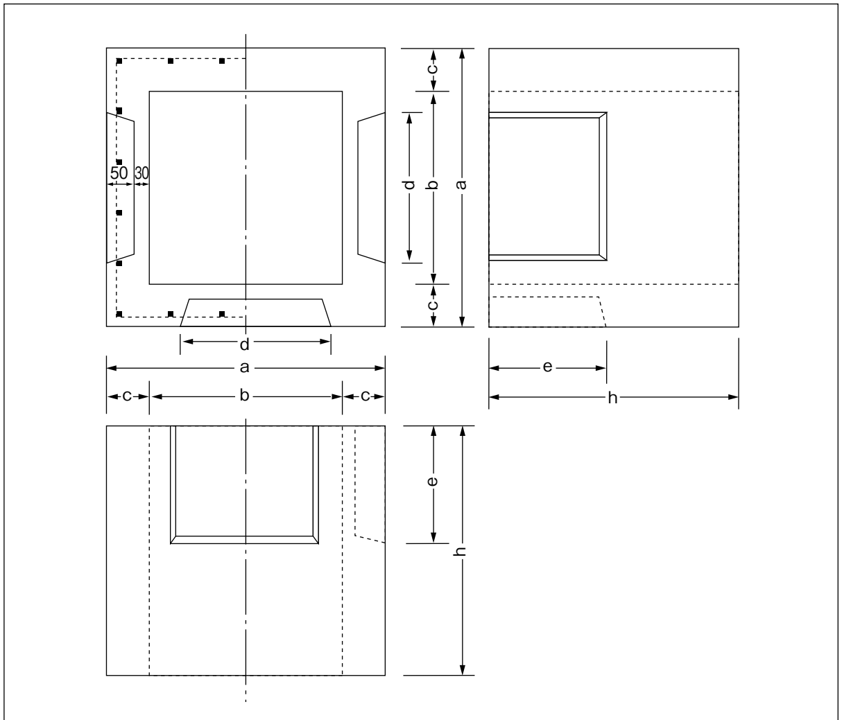
寸法表
