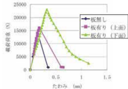
荷重・たわみ曲線
