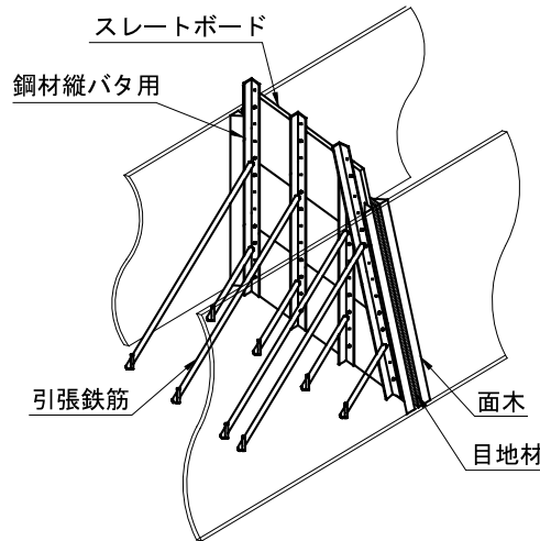
設置完了の模式図
