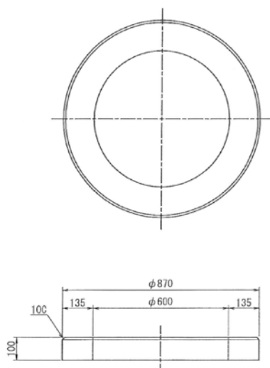
〈ハンドホール用調整リング〉 重量：75kg
