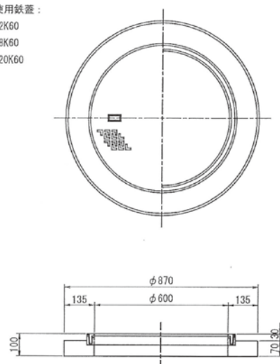
〈ハンドホール用口環リング（アスファルト用）〉 重量：55kg
