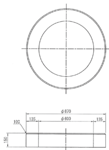
〈ハンドホール用調整リング〉 重量：110kg
