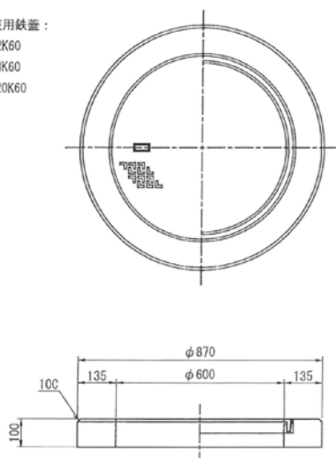
〈ハンドホール用口環リング〉 重量：75kg
