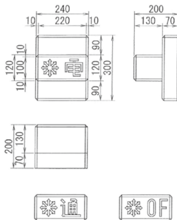
〈MK-A埋設標〉 重量：21kg
