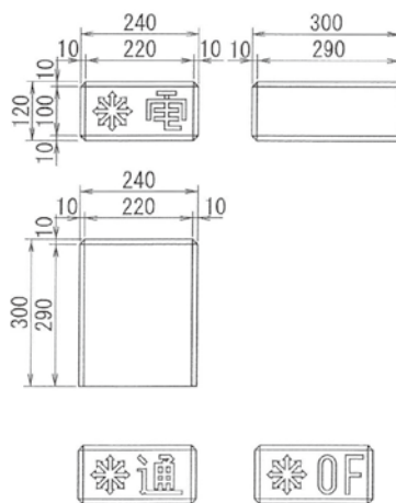
〈MK-D埋設標〉 重量：20kg
