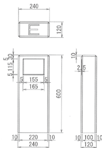
〈MK-E埋設標〉 重量：41kg
