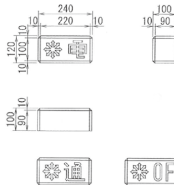
〈MK-B埋設標〉 重量：7kg
