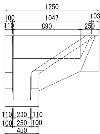
A - A
