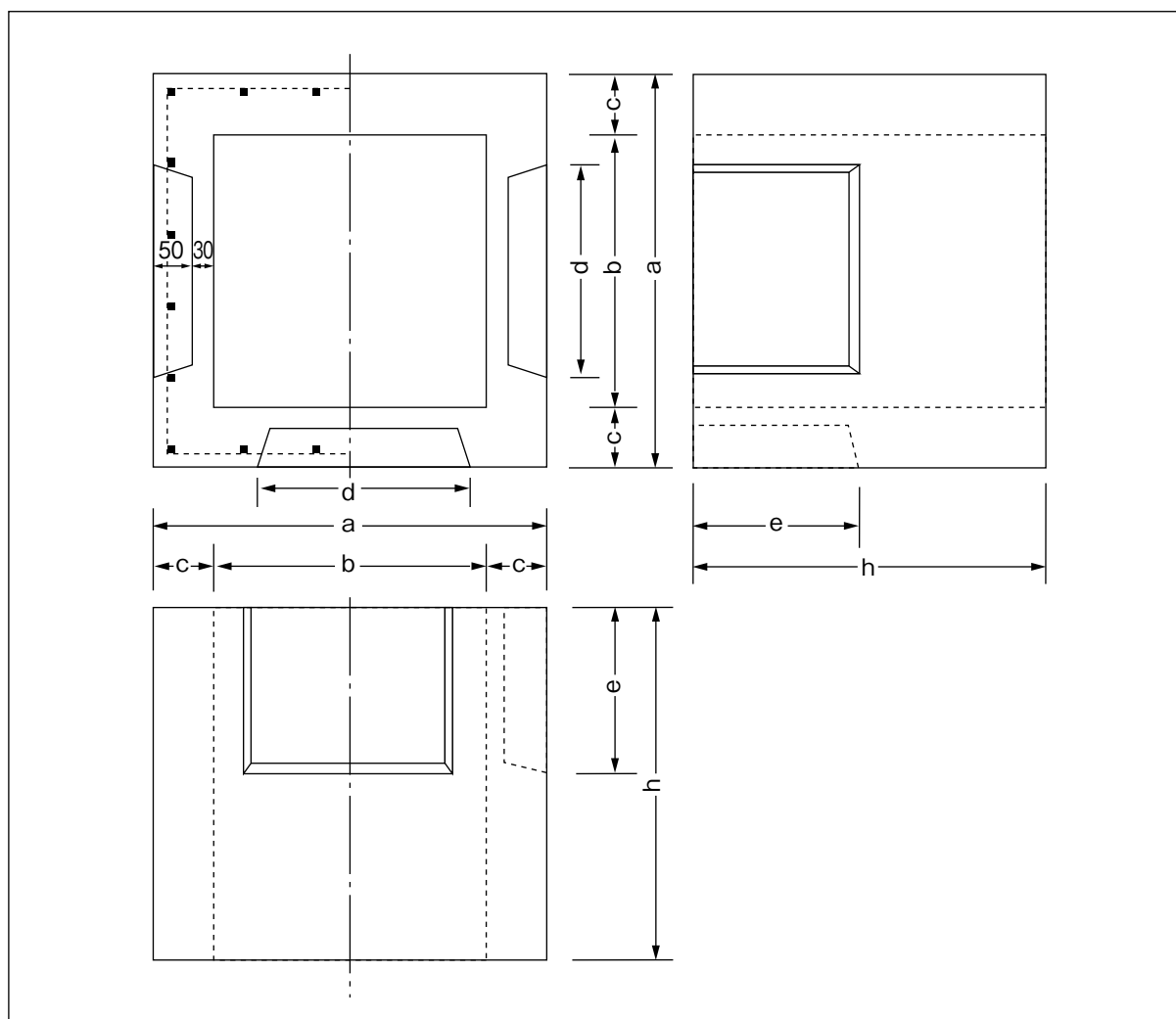
寸 法 表
