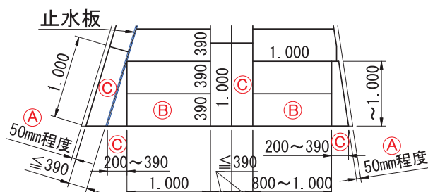
側面図
