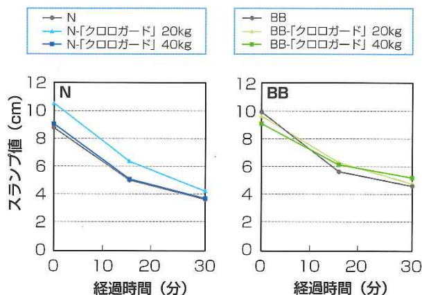
図-2 練上り時のスランプおよびスランプの経時変化の一例（環境温度20℃）
