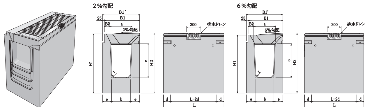
PU3L街渠桝(2%・6%勾配)
