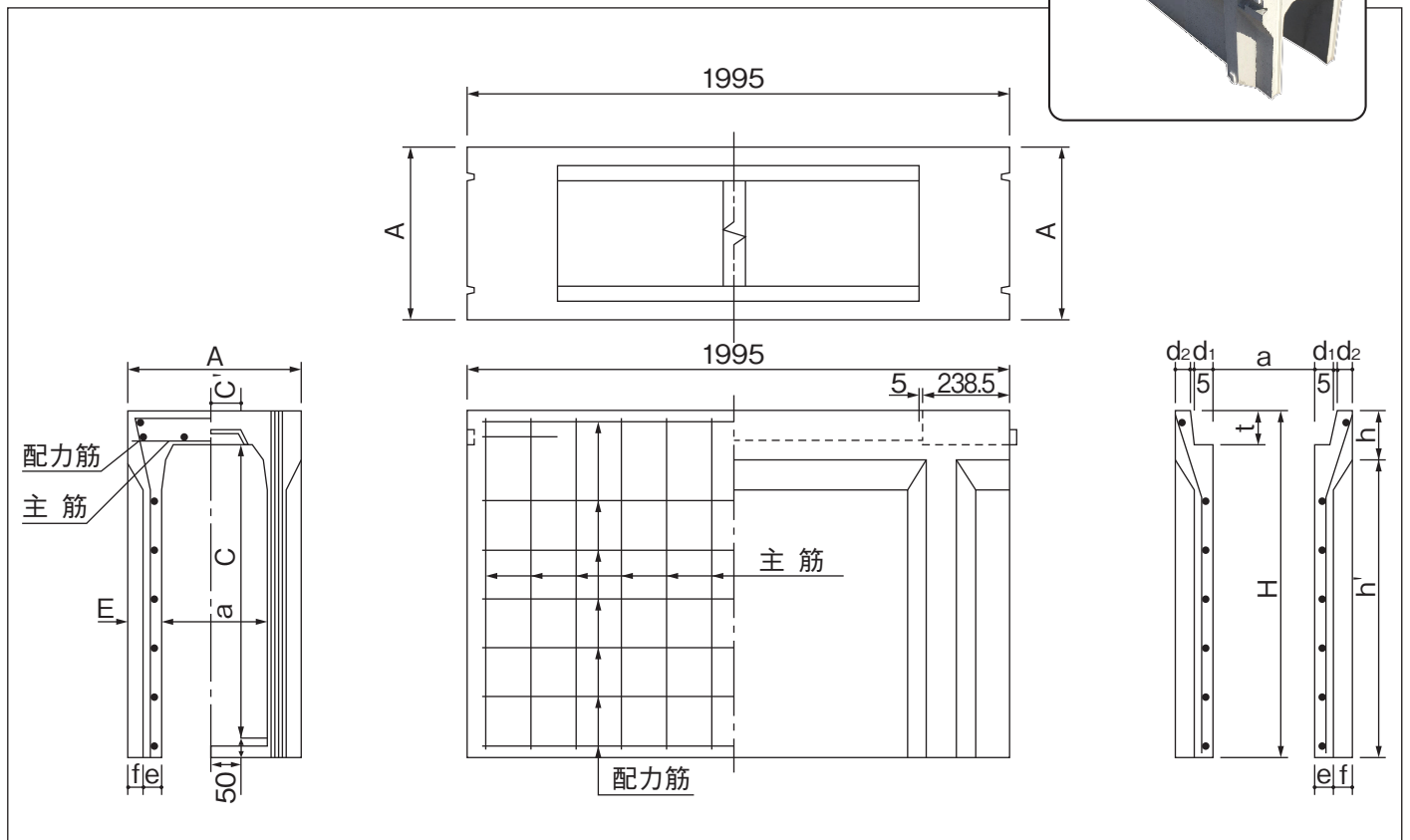
寸法・配筋・重量表
