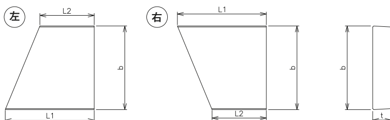
Pu 3 蓋 (落ちふた式U形側溝3種蓋)
