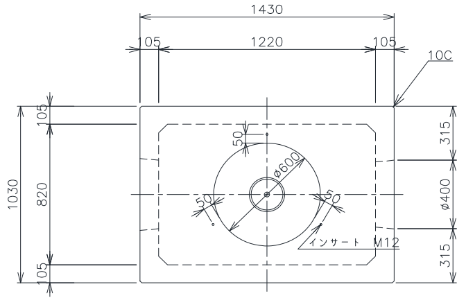
情報ボックス用ハンドホール 800×1200×1000
