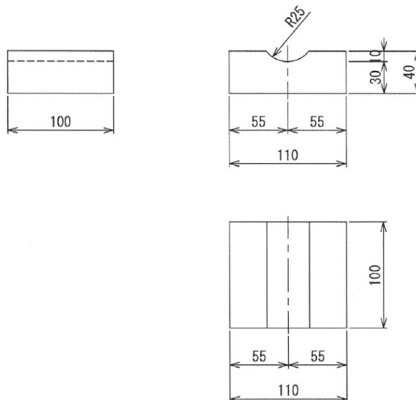
コンクリート製枕木 40A(特)
