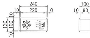
〈MK-B埋設標〉 重量：7kg
