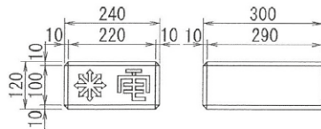
〈MK-D埋設標〉 重量：20kg
