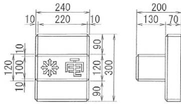
〈MK-A埋設標〉 重量：21kg
