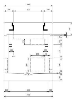
A-A断面図
