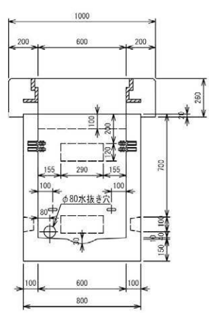
B-B断面図
